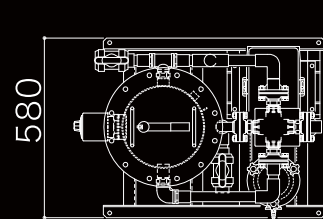
ろ過装置平面図
